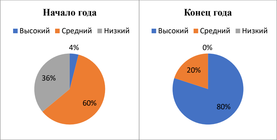
Рисунок 4. Грамматический строй
