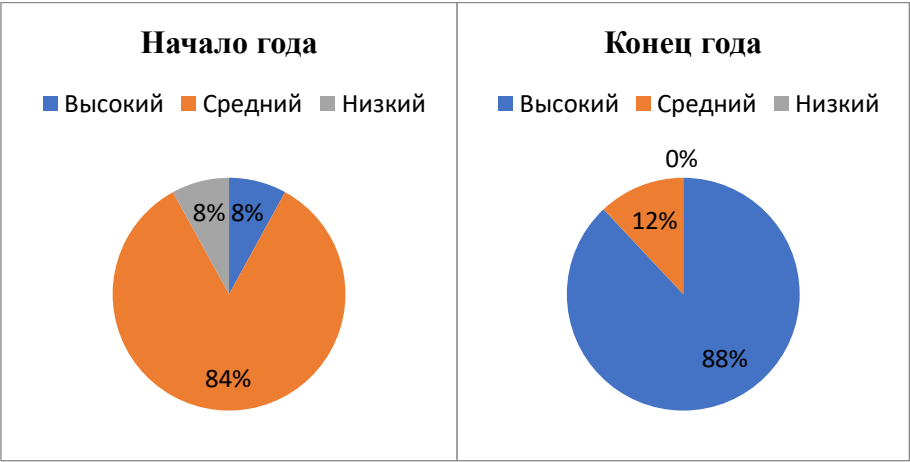
Рисунок 3. Словарный запас
